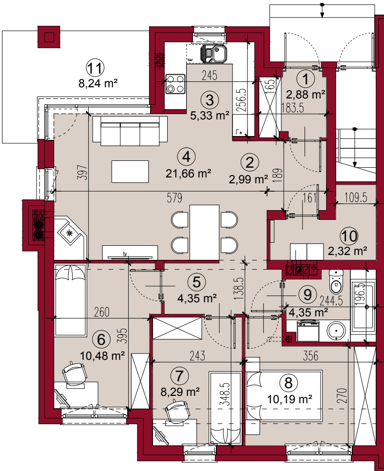
RZUT PARTERU
