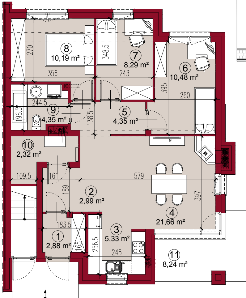
RZUT PARTERU
