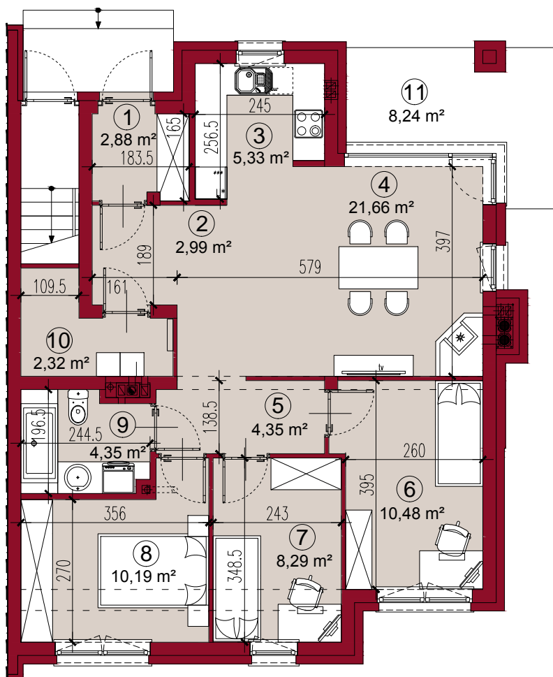
RZUT PARTERU
