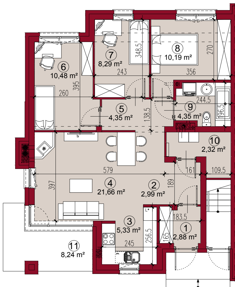
RZUT PARTERU
