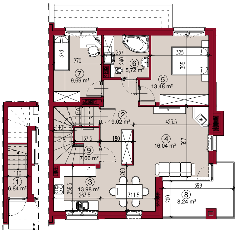
RZUT PARTERU
