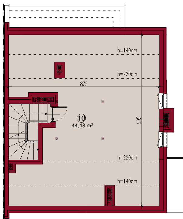
RZUT PODDASZA NIEUŻYTKOWEGO
