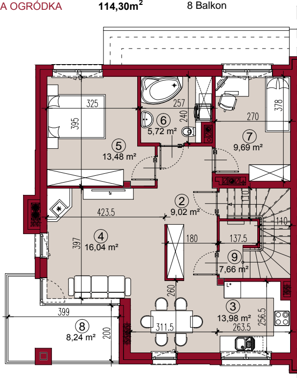
RZUT PIĘTRA
