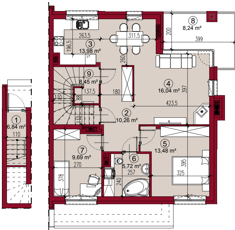
RZUT PARTERU
