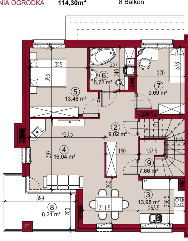
RZUT PIĘTRA
