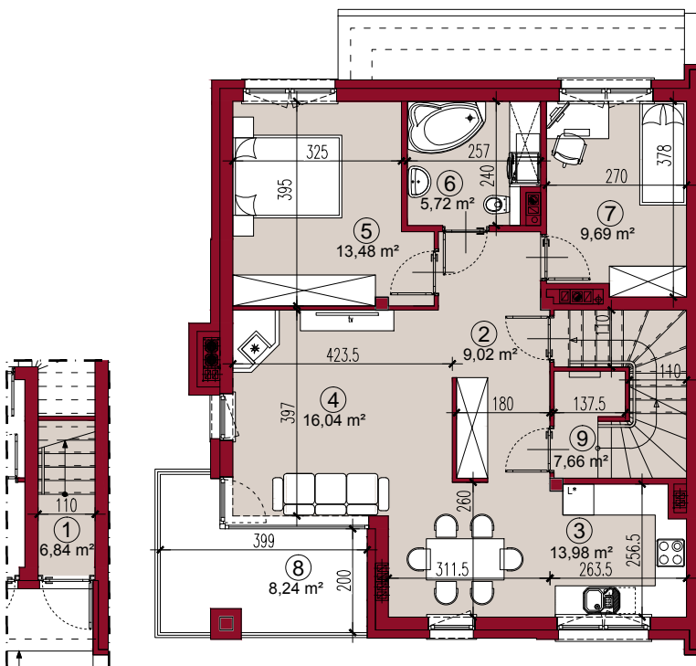
RZUT PARTERU
