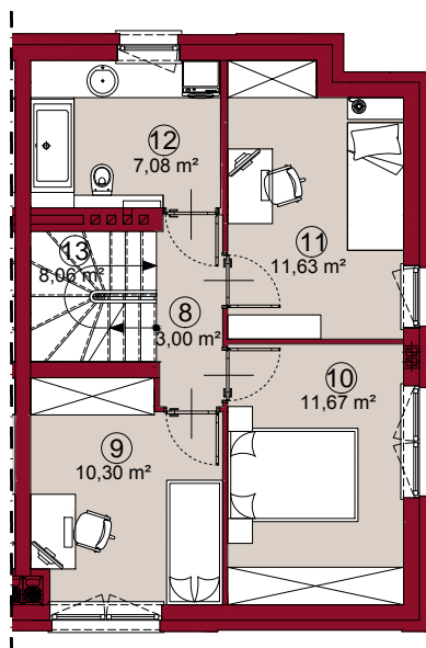
RZUT PIĘTRA
