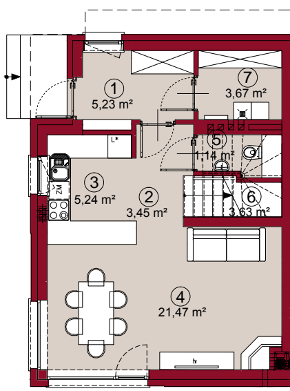
RZUT PARTERU
