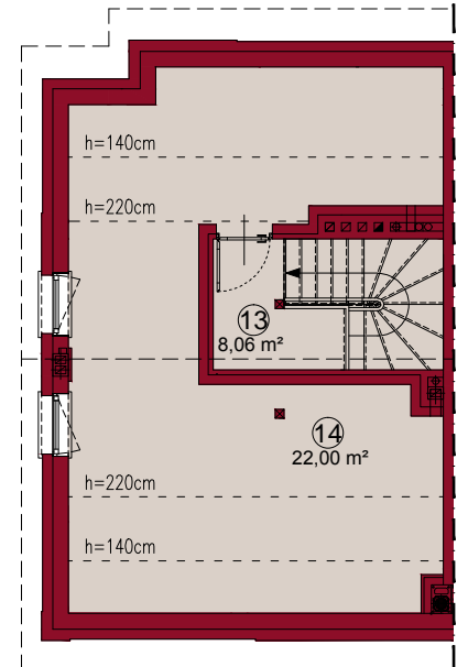
RZUT PODDASZA NIEUŻYTKOWEGO
